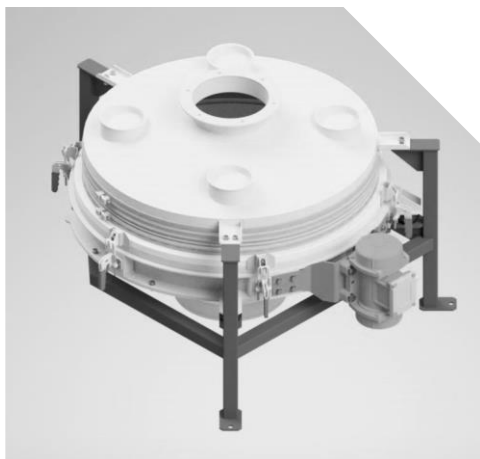
1. ábra Vibrációs kontroll szita modellje
