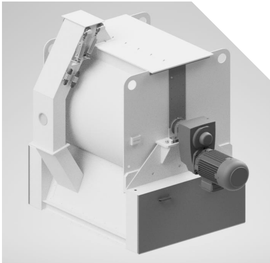
1. ábra Lapatos keverőgép modellje
