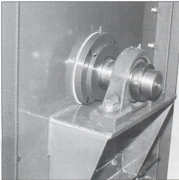
Labirint tömítéssel With labyrinth packing
