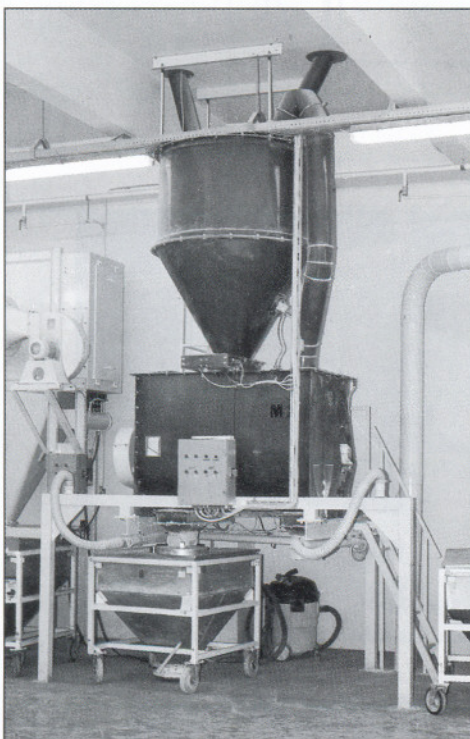
Elő- és utótartállyal With pre- and post-bin
