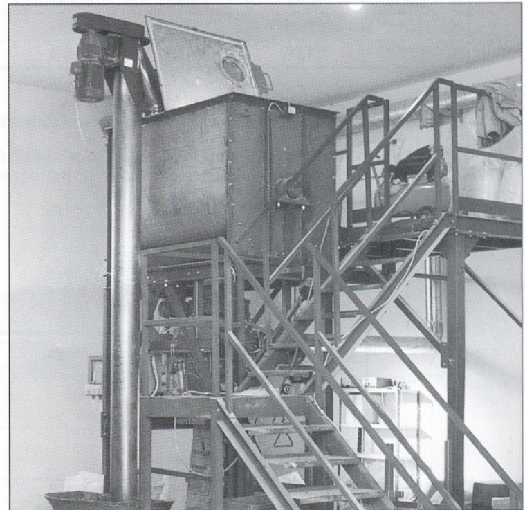
Felhordó csigával, álvánnyal With delivering worm and frame
