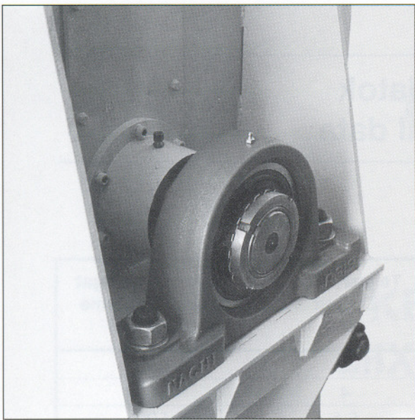
Tömszelencés tömítéssel With stuffing box packing
