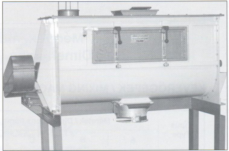
Zsákos ürítővel és tisztítóajtóval With saek discharger, with cleanout door
