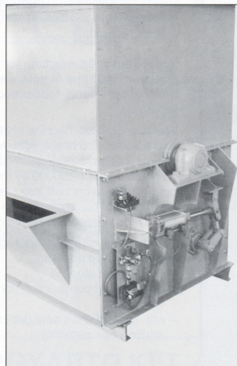
Teljes keresztmetszetű, távvezérelt, pneumatikus ürítőnyílással Of total cross section, remote controlled, with pneumatic discharging hole
