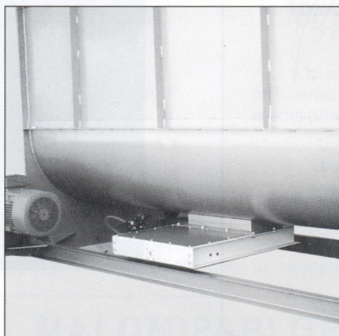
Pneumatikus vagy motoros távvezérlésű tolózárral With gate valve of pneumatic or motorized remote control
